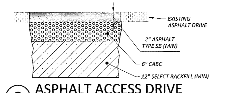
9 ASPHALT ACCESS DRIVE N.T.S.
