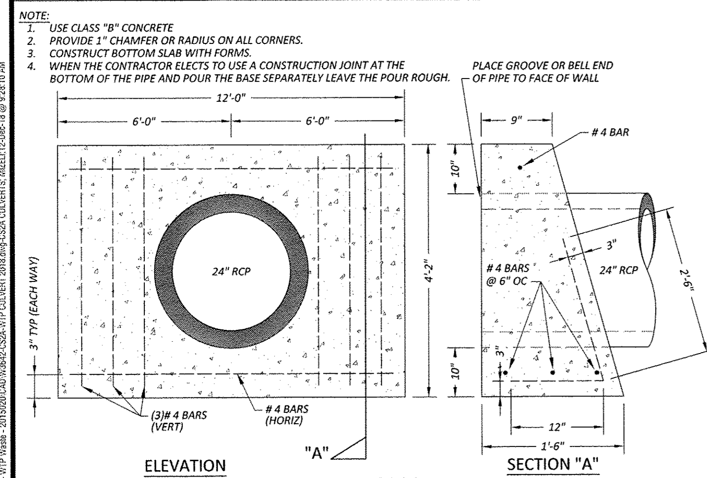
8 HEADWALL N.T.S.
