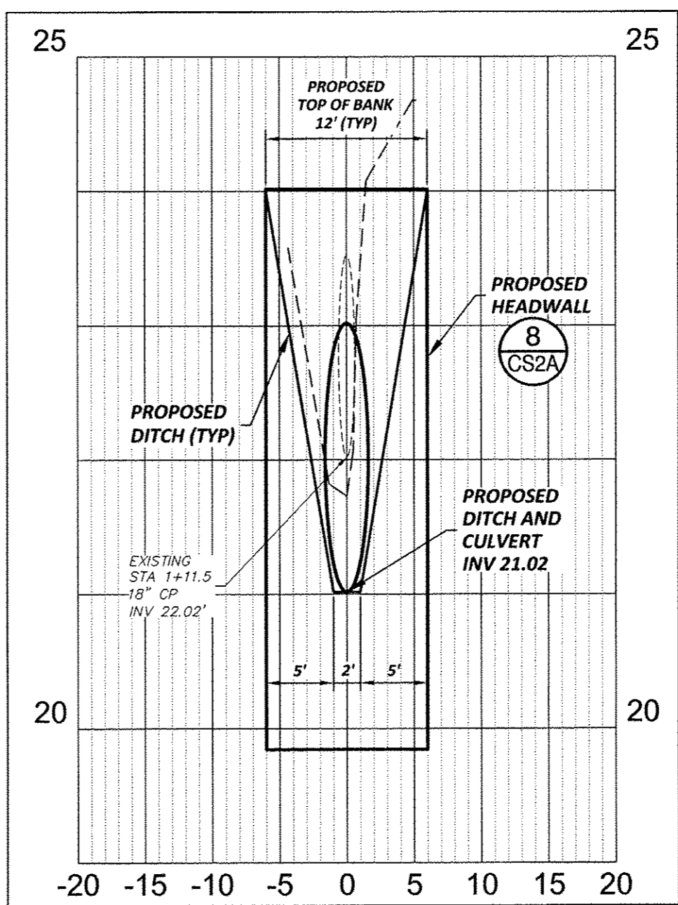
5 SECTIONS - STA 1+11.3 SCALE: 1" = 10'
