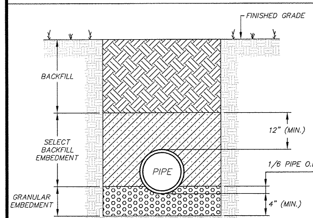
7 CLASS 'C' BEDDING CONC. PIPE N.T.S.
