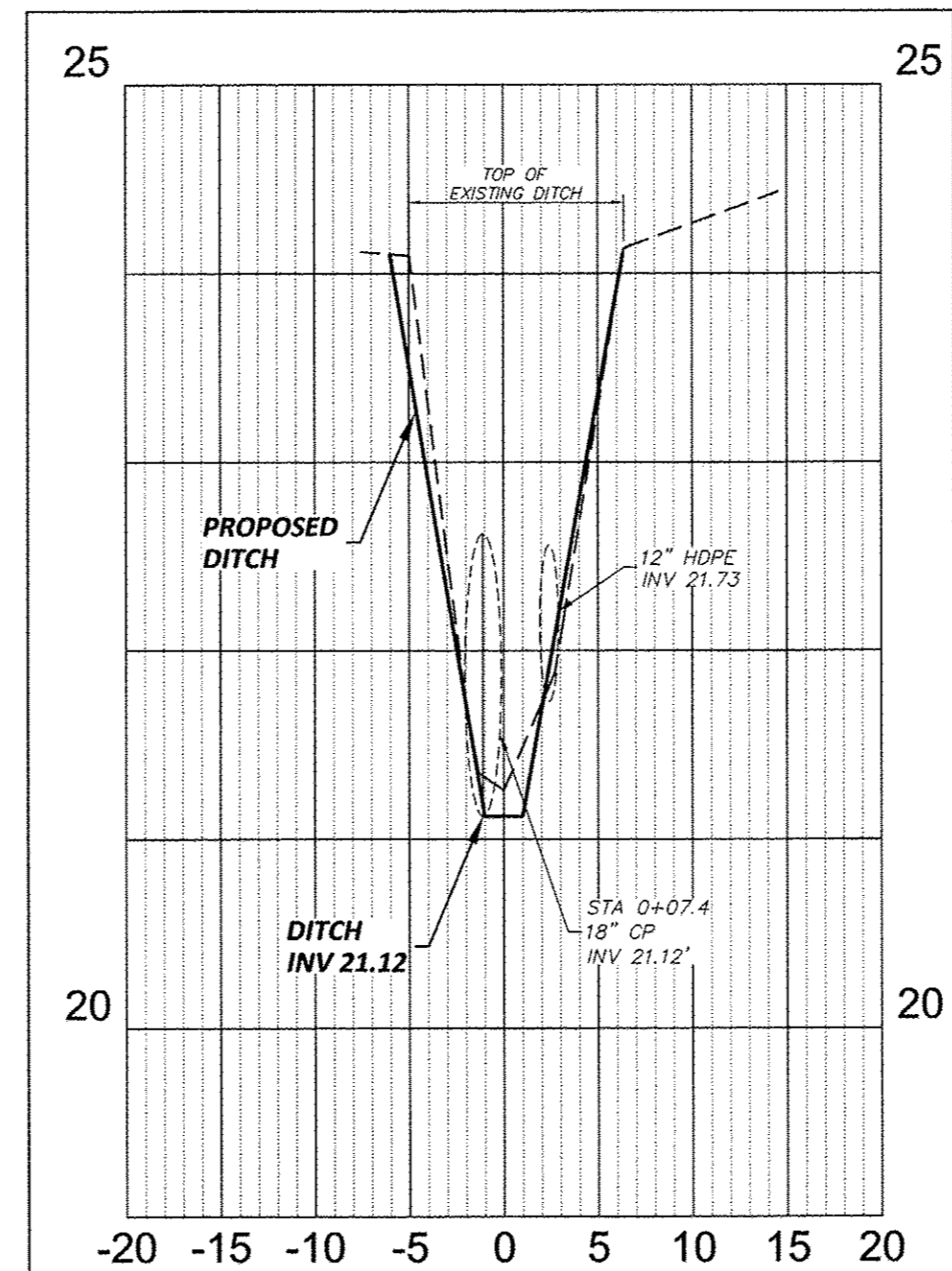
4 SECTIONS - STA 0+08.67 SCALE: 1" = 10'
