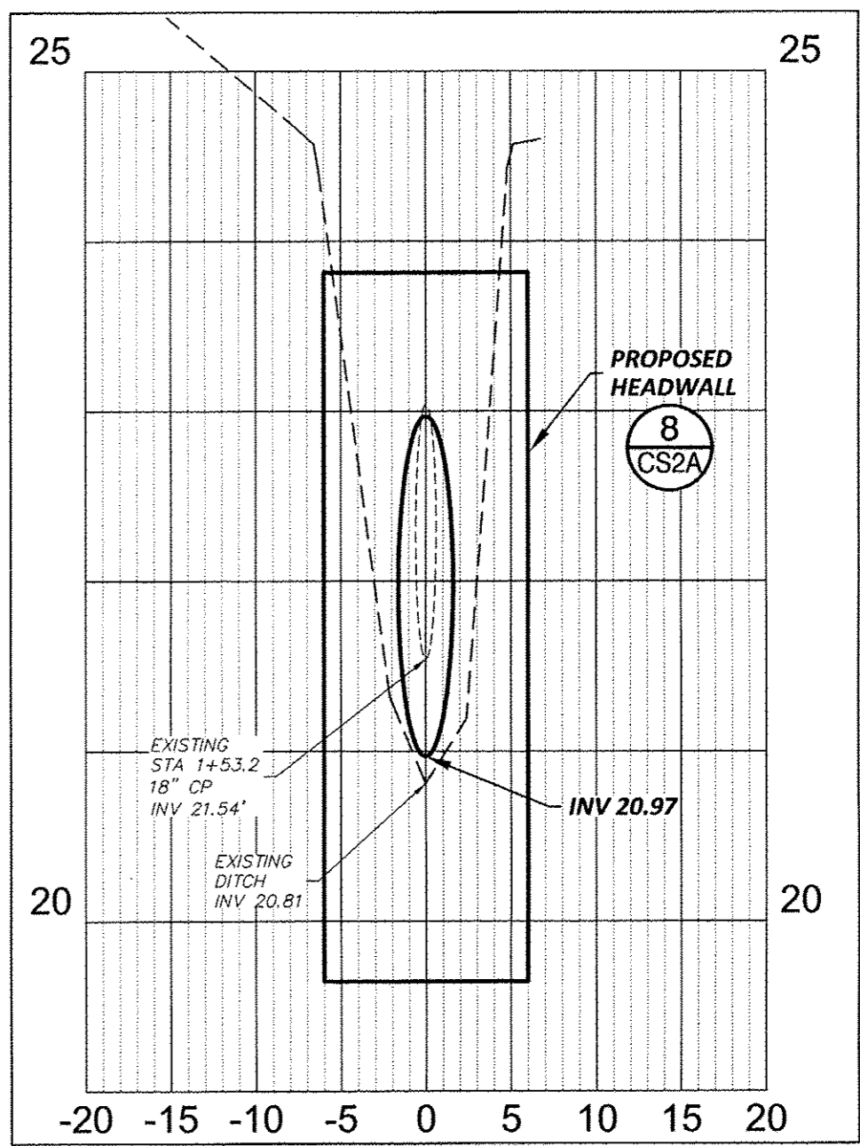
6 SECTIONS - STA 1+60 SCALE: 1" = 10'
