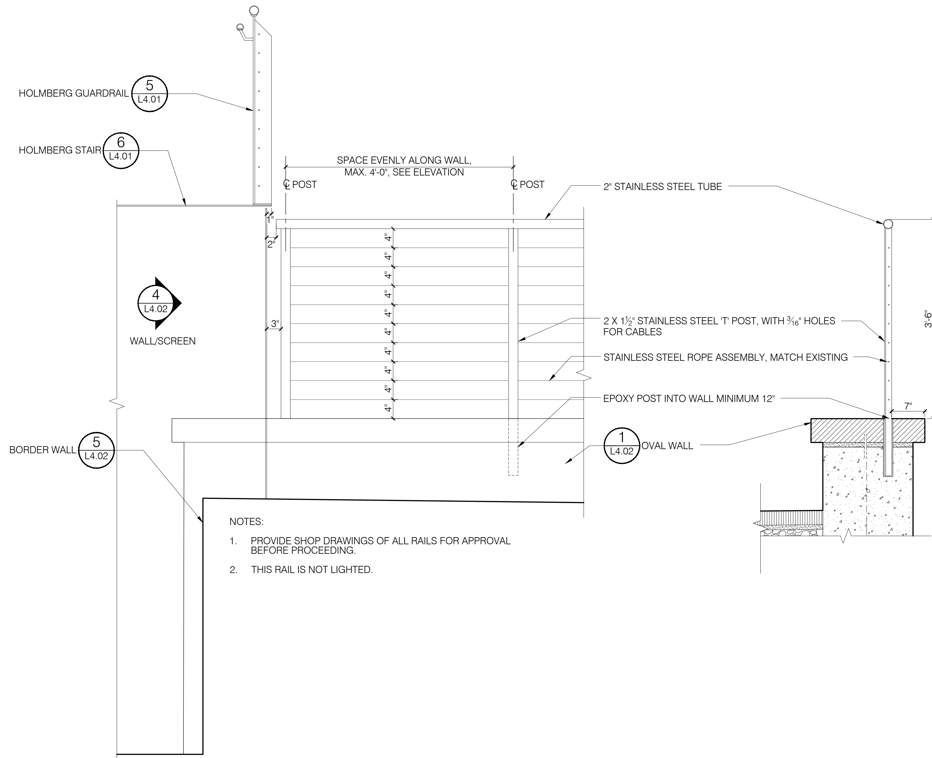
1 OVAL GUARDRAIL - ELEVATION L4.03 SCALE: 1" = 1'-0"
