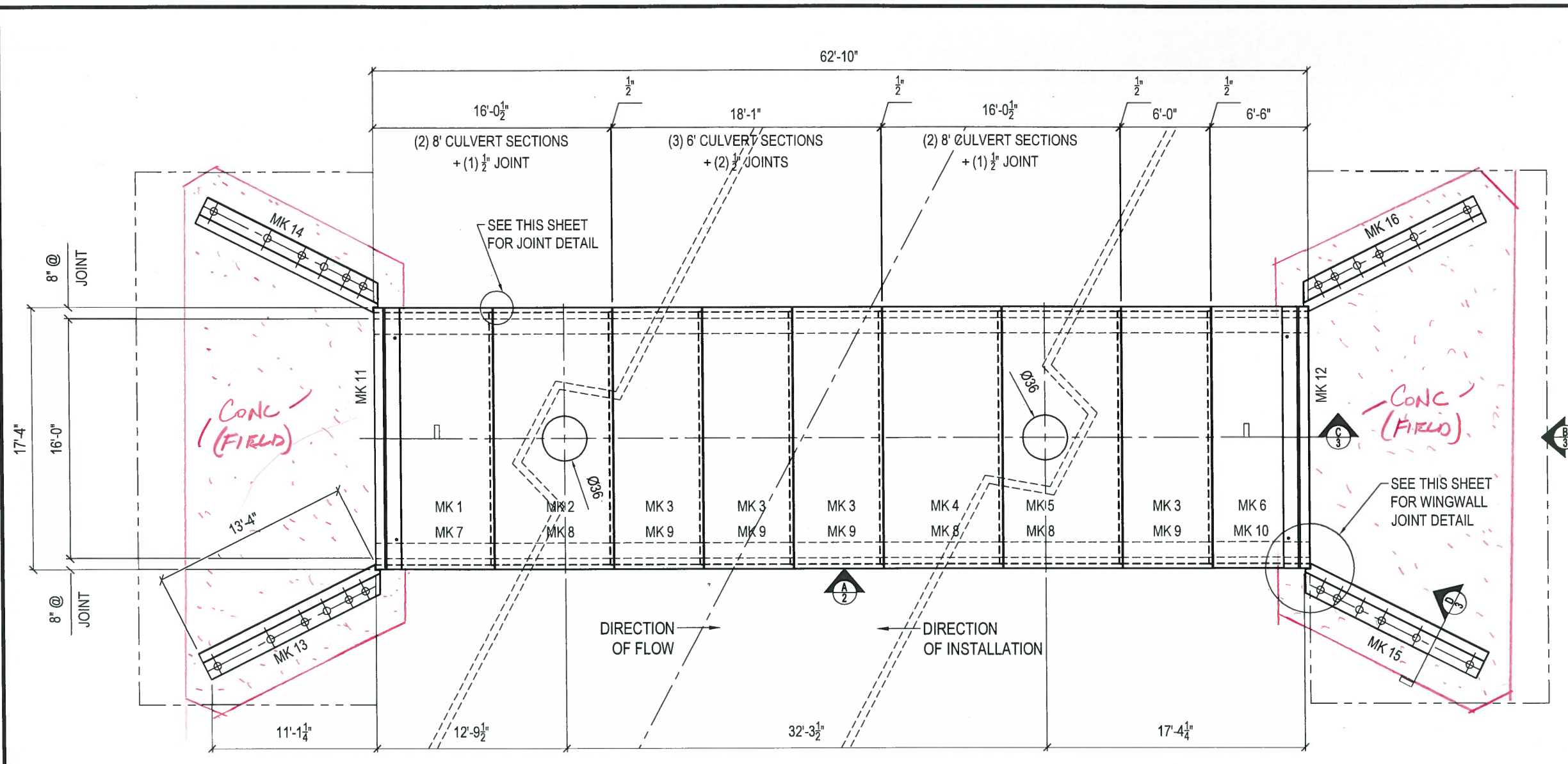
PLAN VIEW SCALE: 1/8" = 1'-0"
