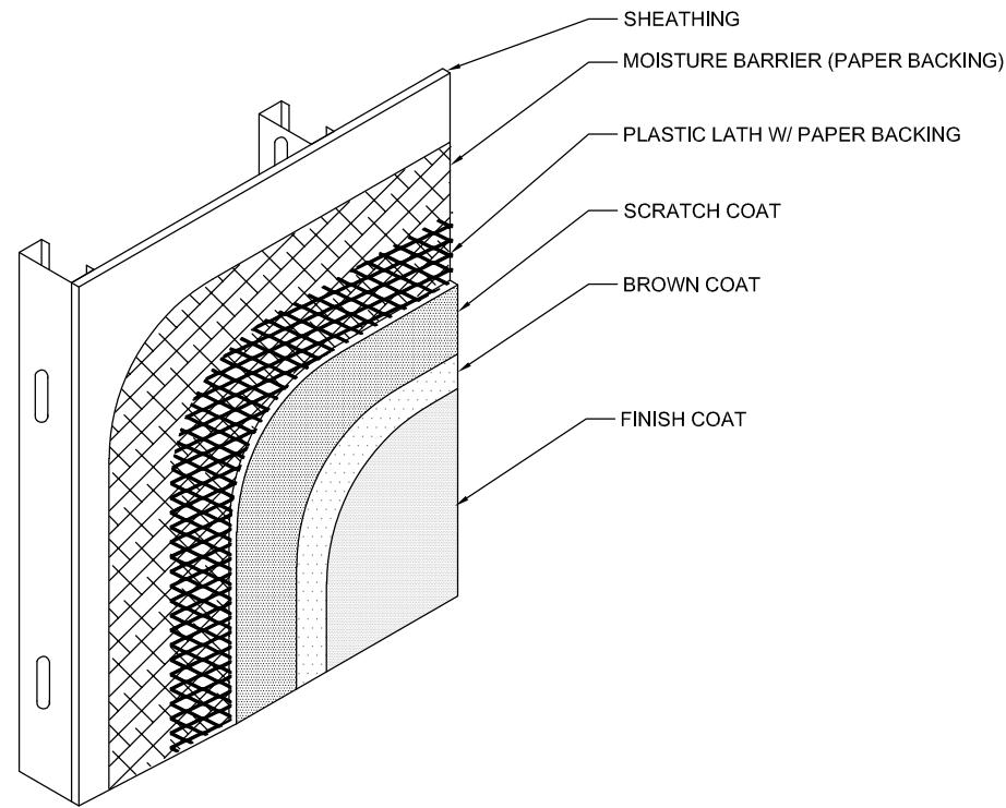
1 STUCCO WALL CLADDING SCALE: NTS
