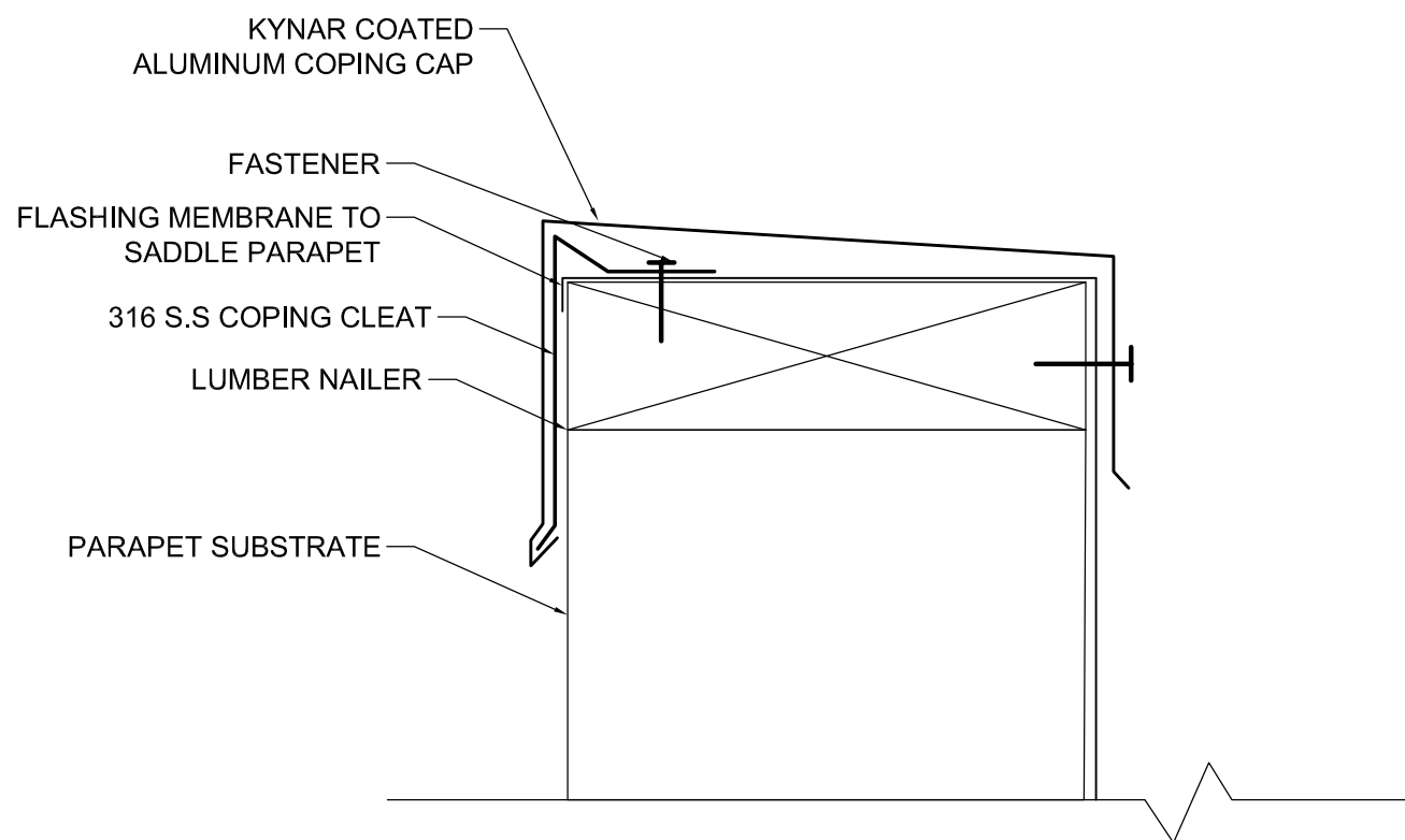
4 COPING CAP & CLEAT SCALE: NTS
