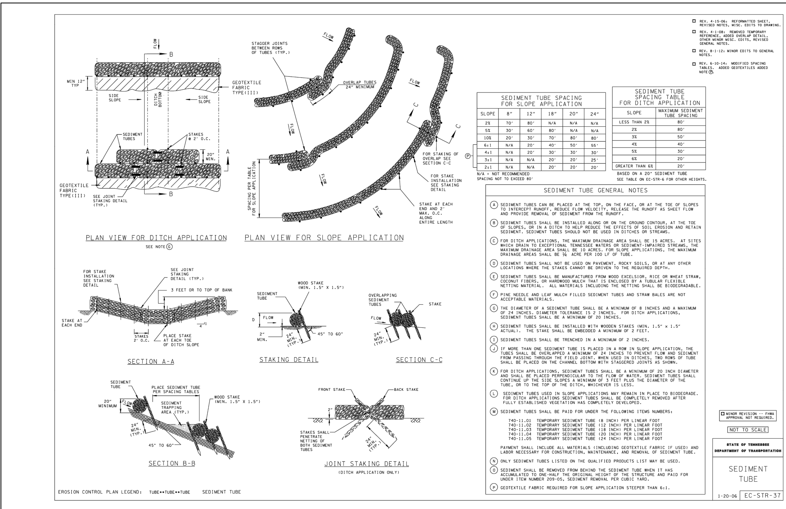
DETAIL 808 SEDIMENT TUBE N.T.S.
