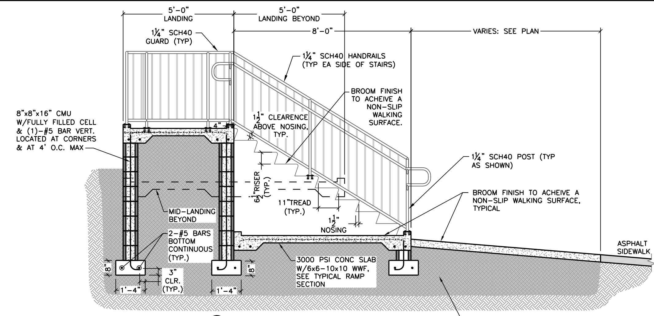
RAMP SECTION SCALE: 3/8"=1'-0"
