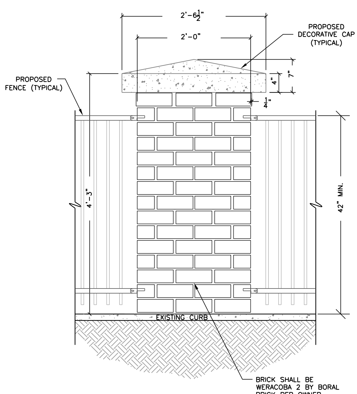
COLUMN ELEVATION SCALE: 1"=1'-0"
