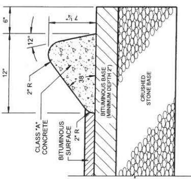
EXTRUDED 6" SLOPING CONCRETE CURB SEE NOTES (L) & (D)
