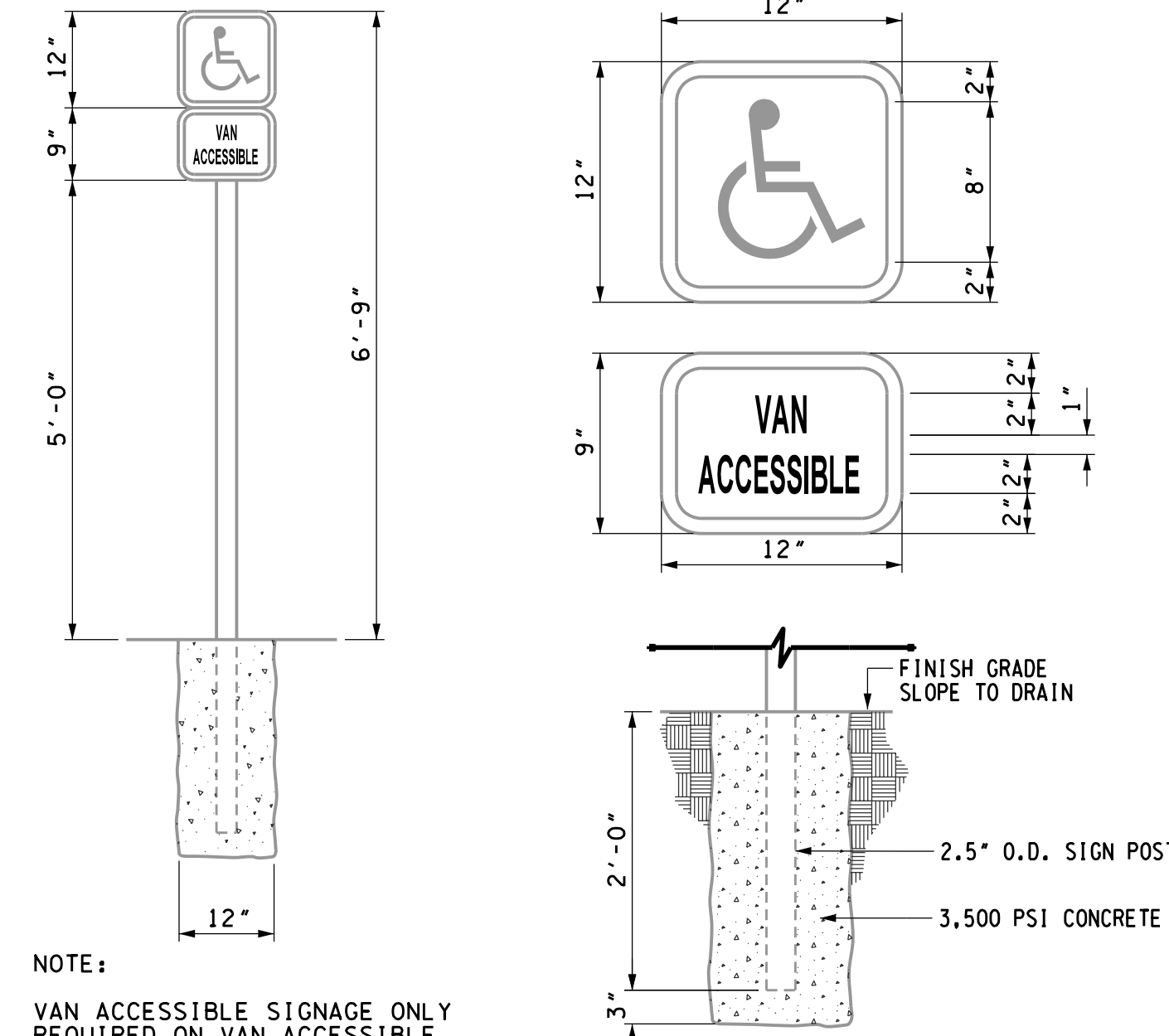
HANDICAP SIGN DETAIL N.T.S.
