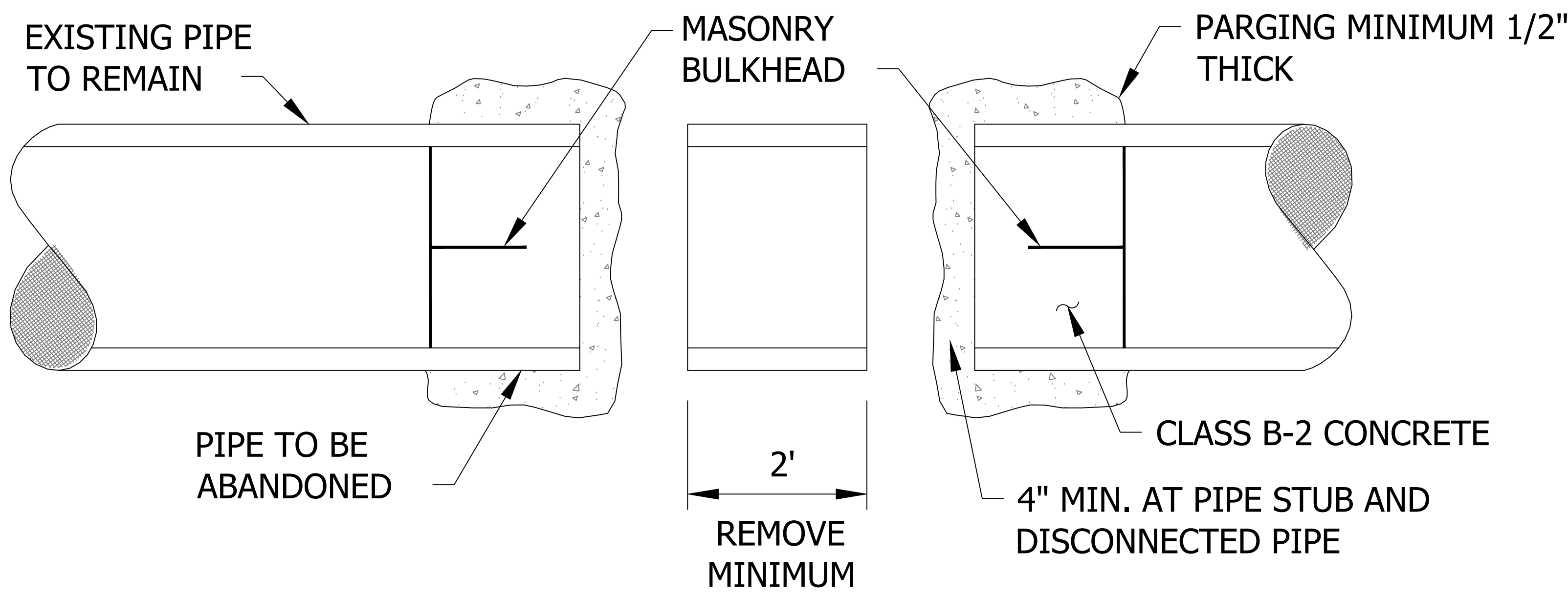
PIPE ABANDONMENT N.T.S.
