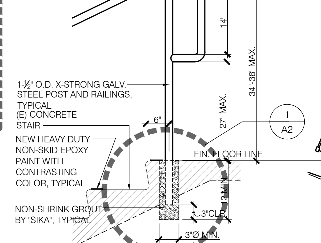
7 SECTION HANDRAIL SCALE: 1" = 1'-0"
