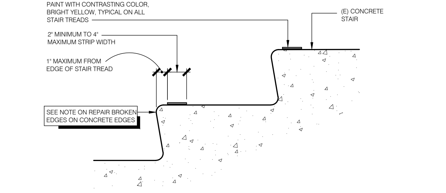
2 EXISTING STAIR TREAD SECTION SCALE: 3" = 1'-0"
