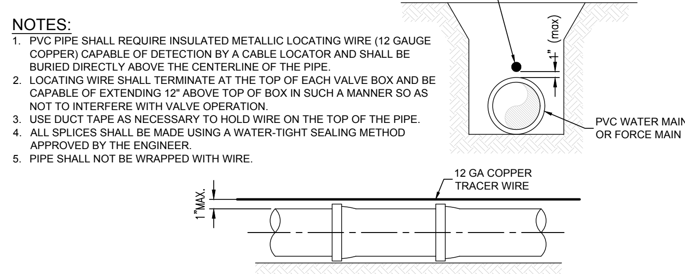
DETAIL PVC PIPE LOCATING WIRE DETAIL SCALE: N.T.S.
