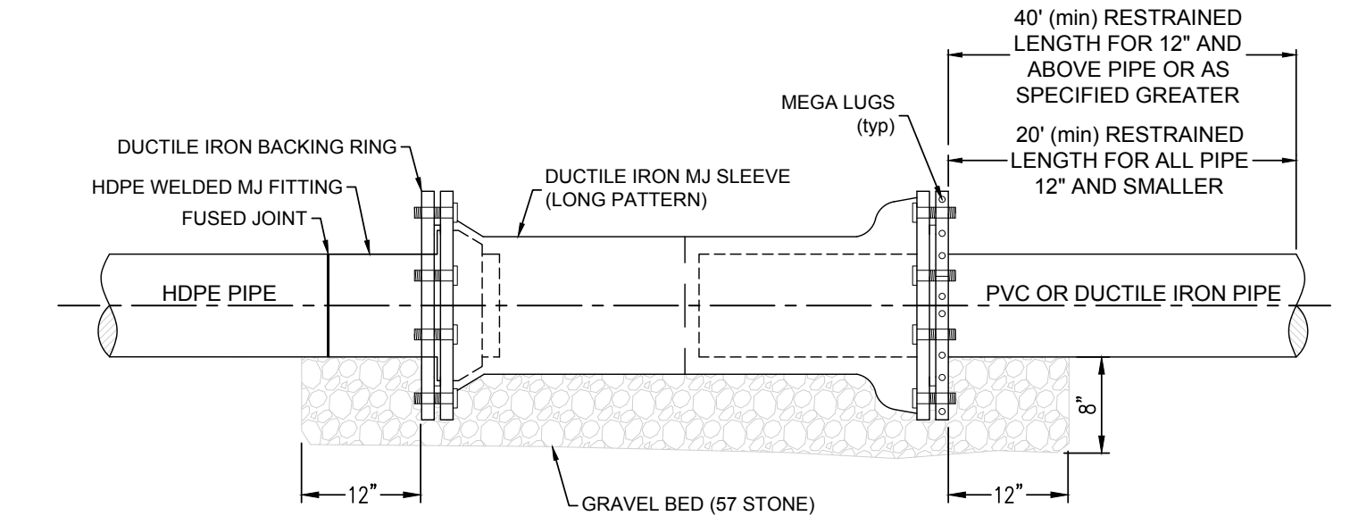
DETAIL HDPE TRANSITION CONNECTION SCALE: N.T.S.
