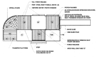
1 BEAUFORT PLAYHOUSE - PLAN SCALE: 1/8"=1'-0"
