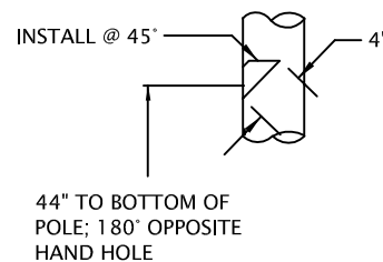
CONDUIT ENTRANCE DETAIL NOTE 1
