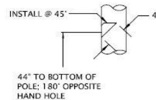
CONDUIT ENTRANCE DETAIL NOTE 1
