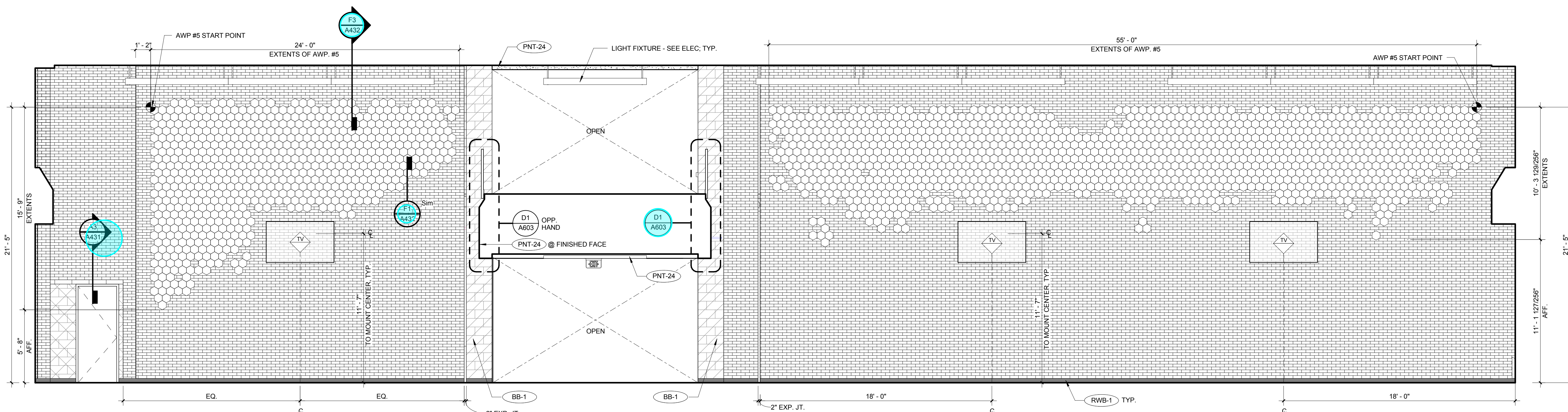
A5 A150 EAST 1/4" = 1'-0" REFERENCED ON A4 / A111A
